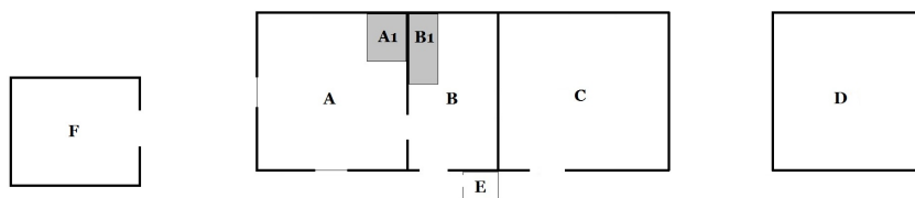
Obr. 9.8: Pôdorys domu Štefana Timuru v osade Baranie. A - Obytná časť, A1 - pec, B - priklet, B1 - pahrutka, C - maštaľ, D - senník, E - chlievik, F - sypanec.
