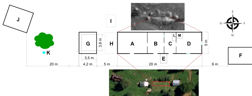
Obr. 9.25: Náčrt rozostavenia a účelu stavieb v usadlosti Andreja Blaščáka, Baranie. Odhadovaný stav v 70. rokoch. A - stodola, B - maštaľ, C - priklet, D - obytná izba, E - chlievik, F - sypanec, G - senník/maštaľ, H,I - dolok, J - stodola, K - prameň pod bukom, L - pahrutka, M - pec. V teréne zamerala Janka Porubská. Pre porovnanie letecký záber z roku 2016. © mapy.cz a záber z roku 1949 © Historická ortofotomapa © GEODIS SLOVAKIA, s.r.o. a Historické LMS © Topografický ústav Banská Bystrica
